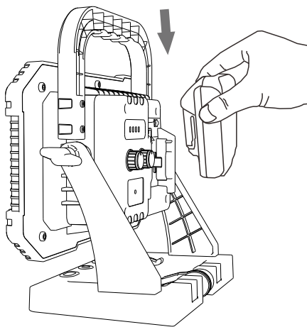
装着時：バッテリーを上方向から差し込んでください
