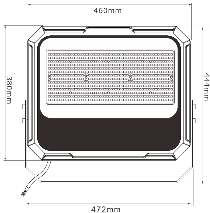
寸法図
