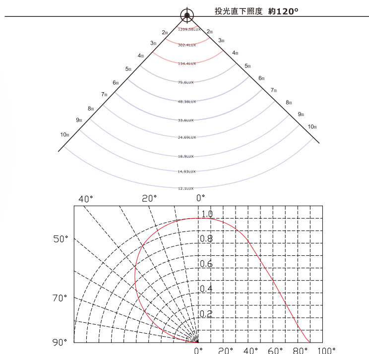
照度分布図面
