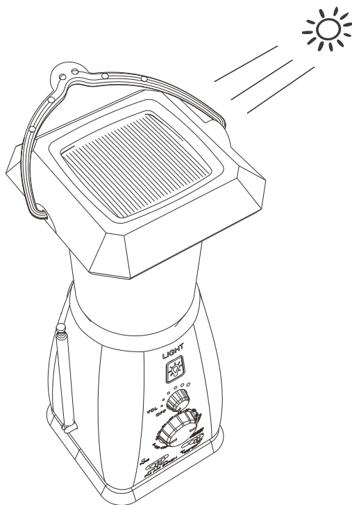
ソーラーパネルで充電：5.5V/35mAh (20000lux太陽光直射)
