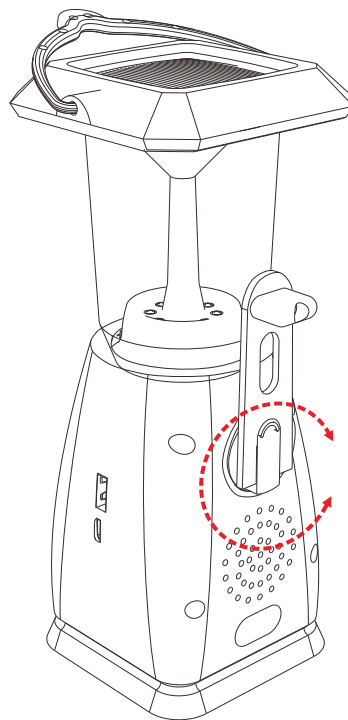
手回しハンドルで充電：5.5V/200mAh (140回転/分の速度)
