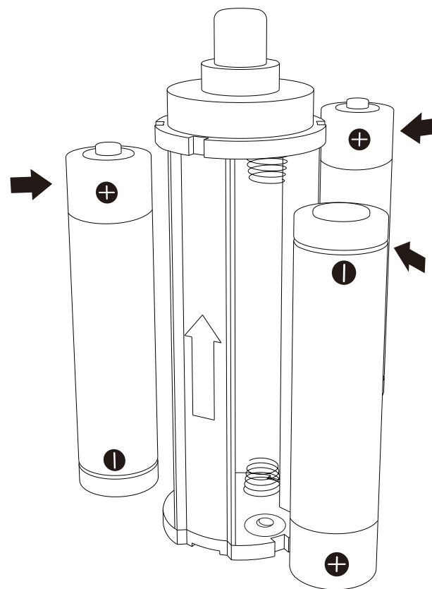
バッテリーカートリッジに乾電池*3本をセットする。
